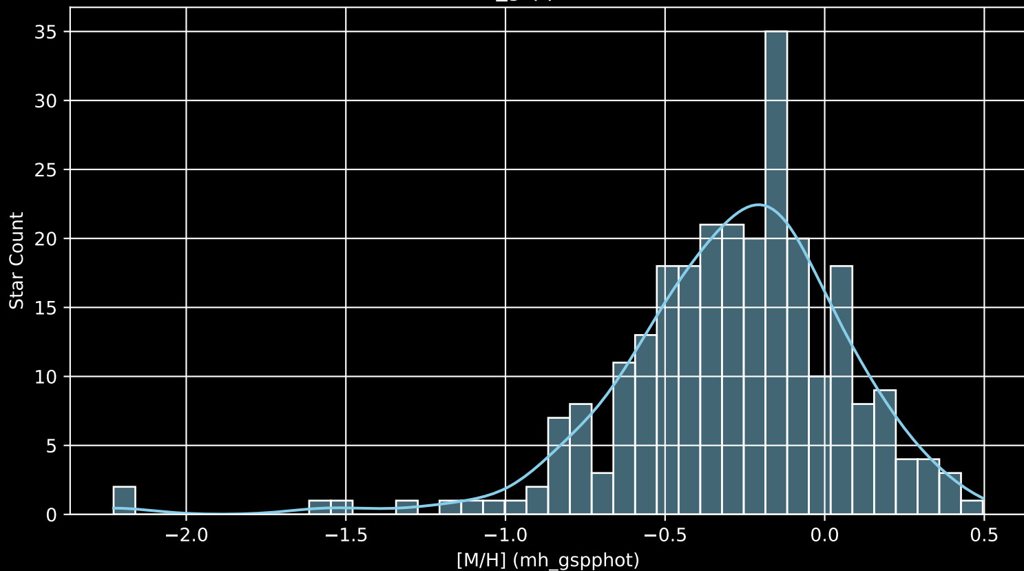
GALAH DR4 Field: [88] [M/H] (mh_gspphot) (n= 263)
