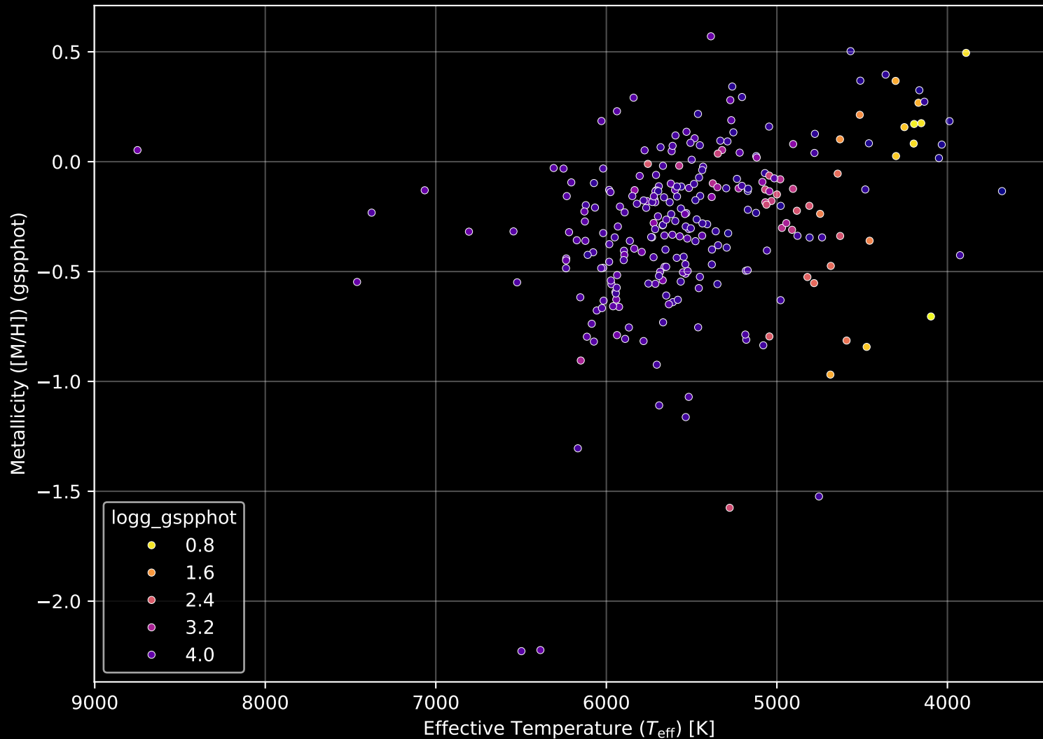
GALAH DR4 Field: [88] Stellar Population Parameters (n= 265)
