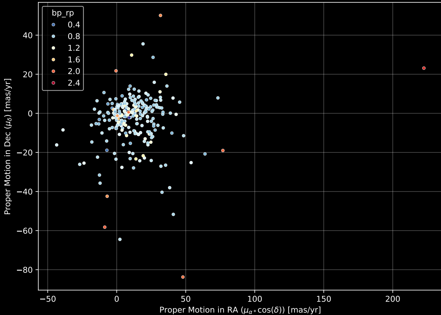
GALAH DR4 Field: [88] Proper Motion Diagram (n= 265)
