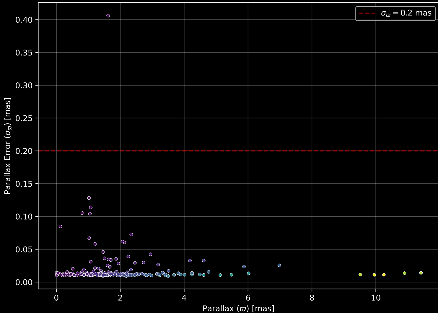
GALAH DR4 Field: [88] Parallax Quality (n= 265)
