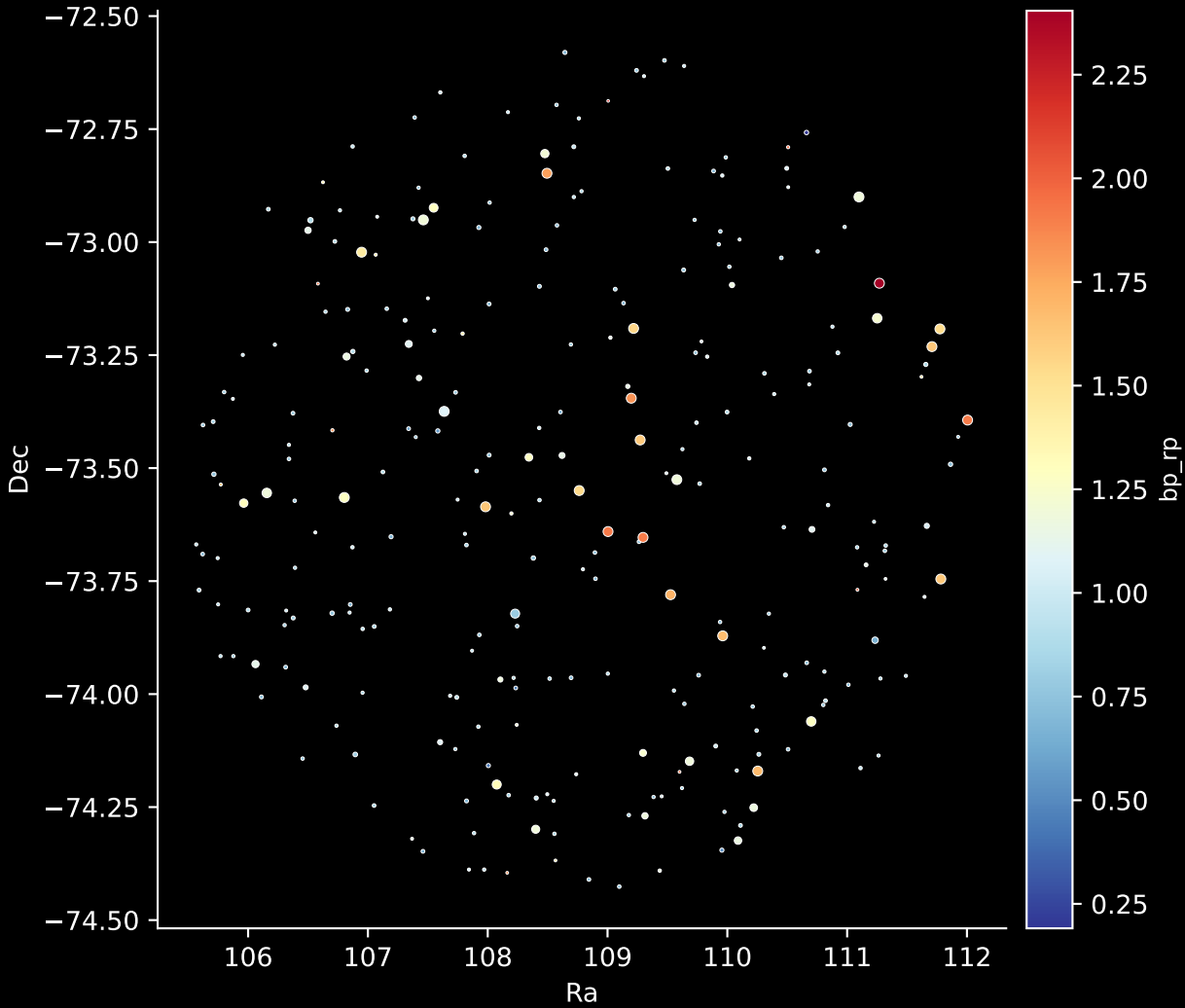
GALAH DR4 Field: [88] Stars: 265
